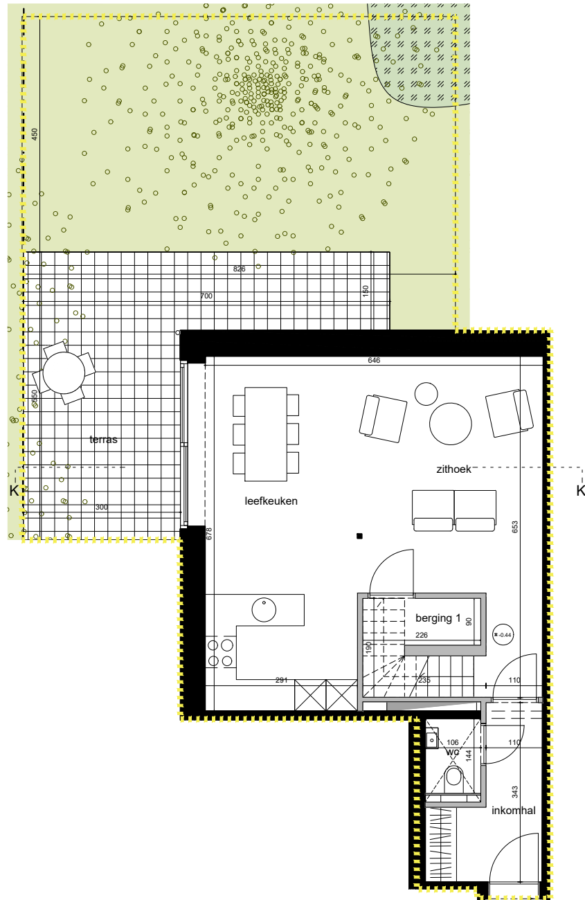
NIVEAU +0
