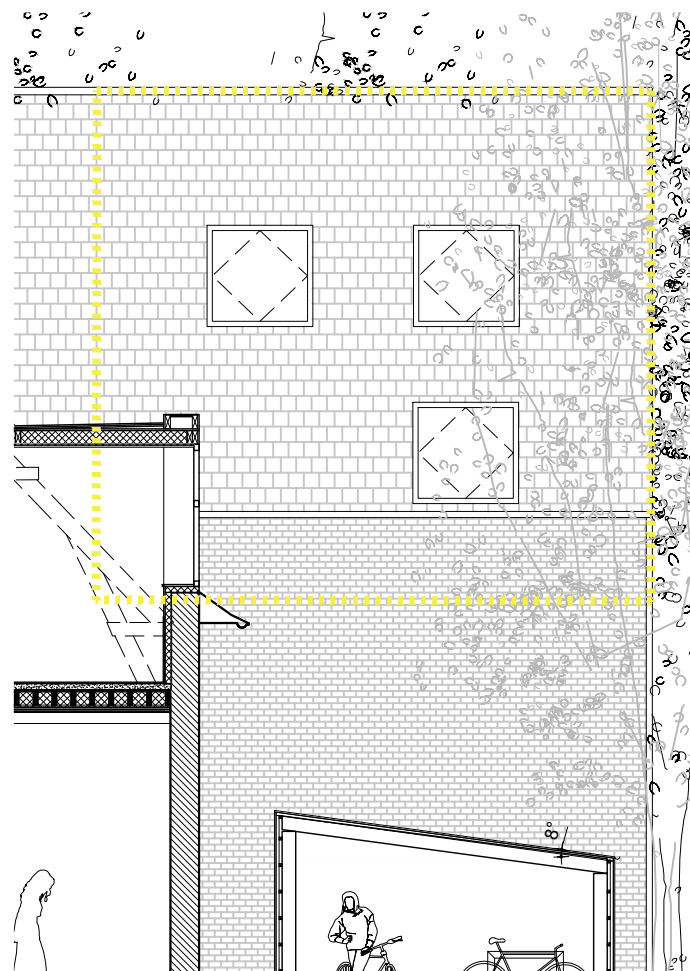
OOSTGEVEL
