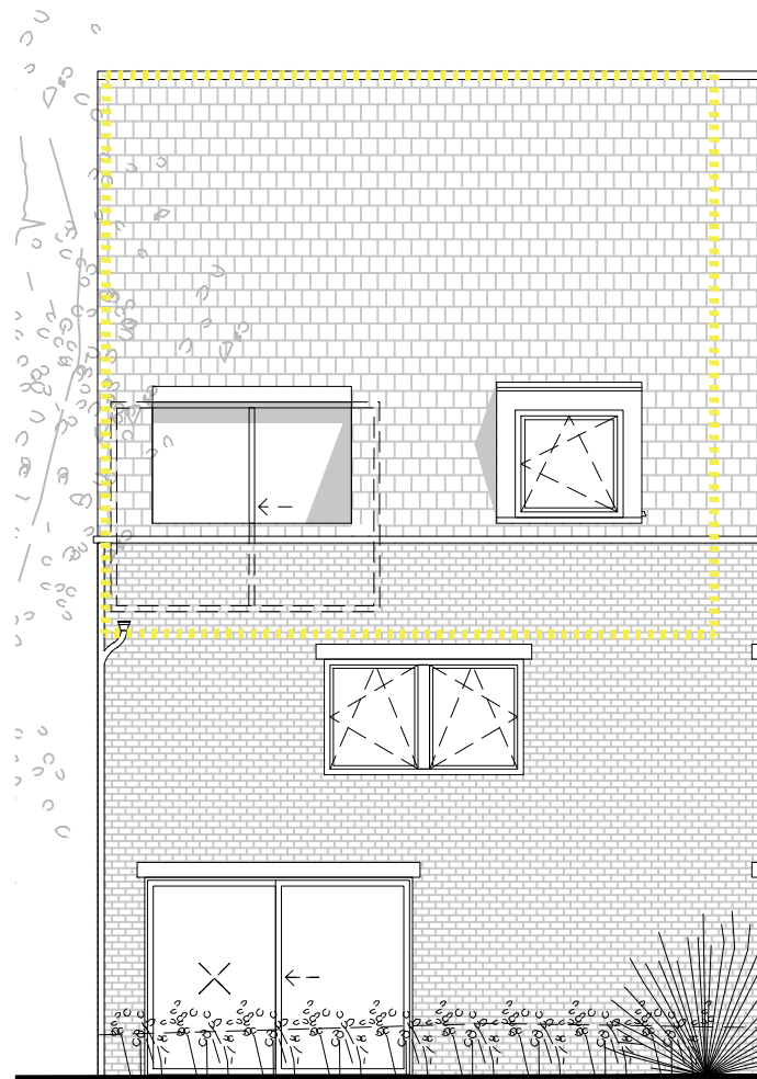
OOSTGEVEL
