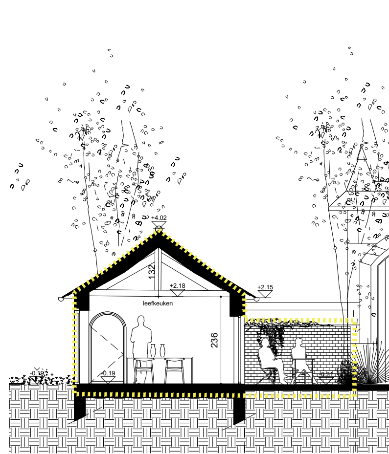
SNEDE DD'
