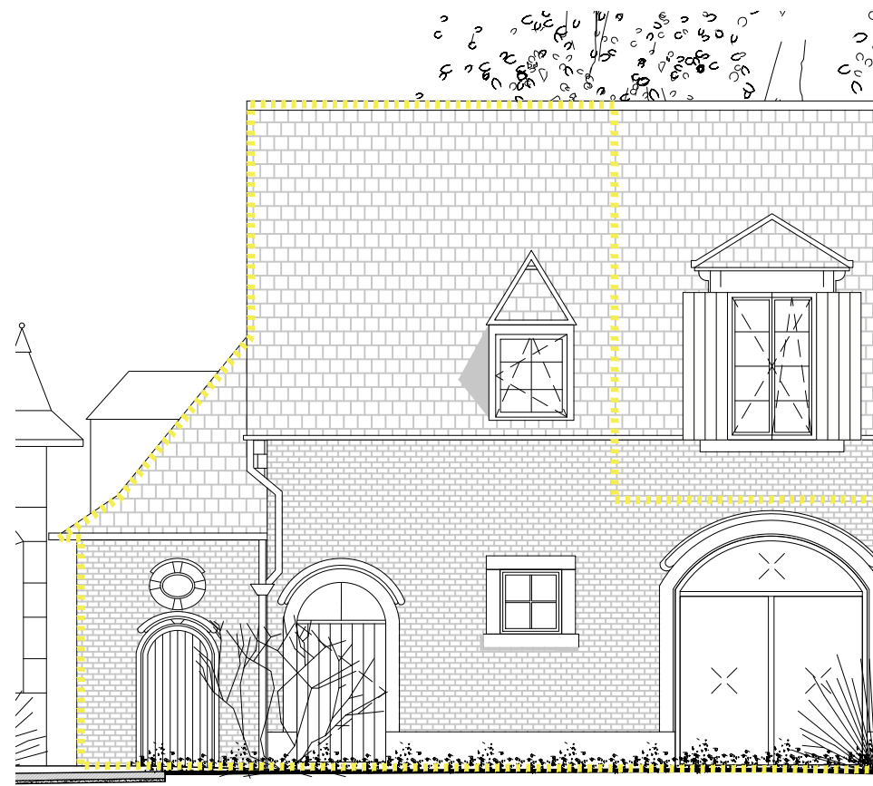
OOSTGEVEL
