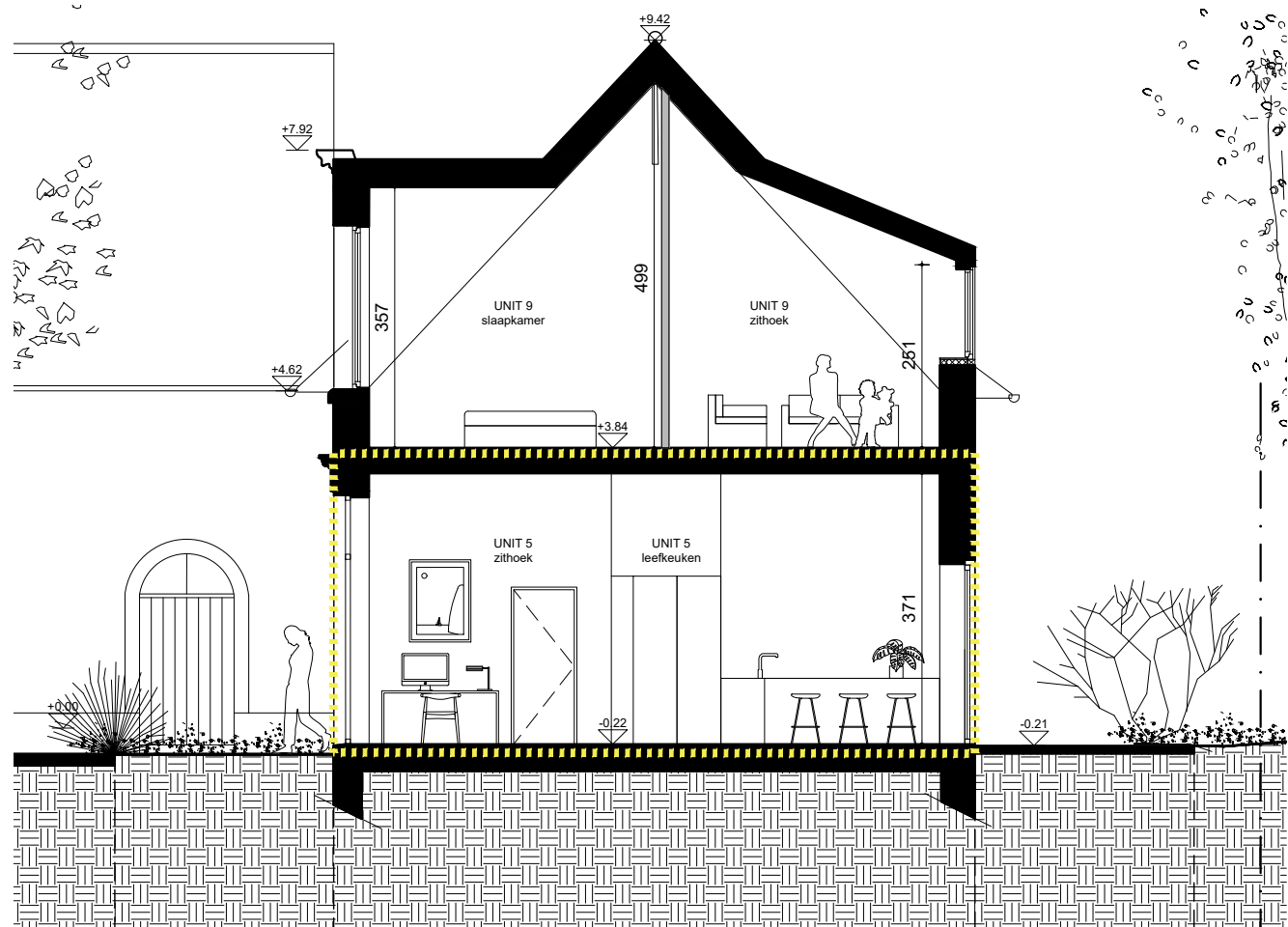
SNEDE NN'
