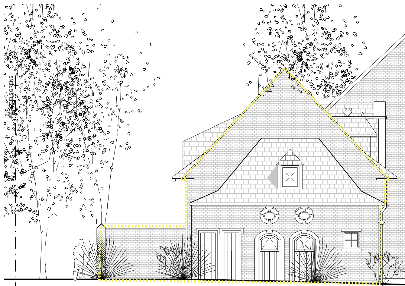
ZUIDGEVEL
