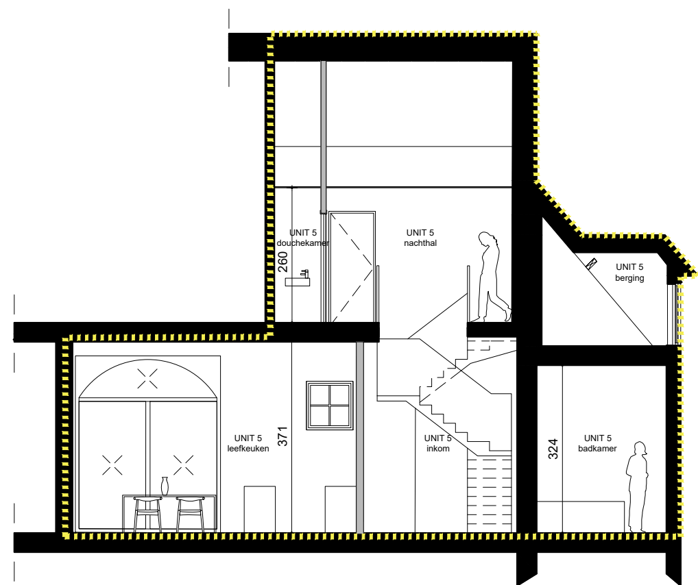
SNEDE PP'
