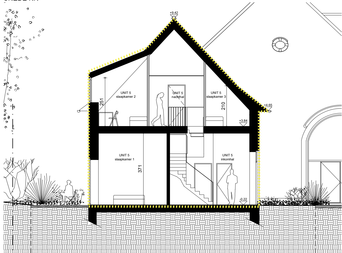
SNEDE NN'
