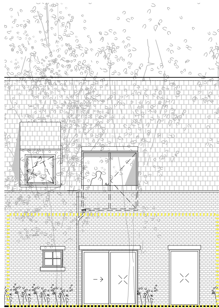
WESTGEVEL
